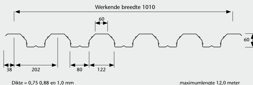
Profiel en afmetingen (mm)
