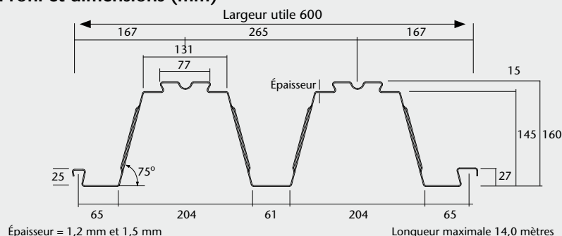
Profil et dimensions (mm)
