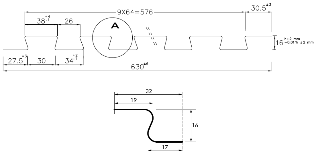
Fig. 1: Dimensions des Profilés à queue d'aronde® Lewis®
