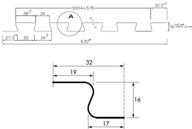
Fig. 1: – Dimensions des profilés à queue d'aronde Lewis®
