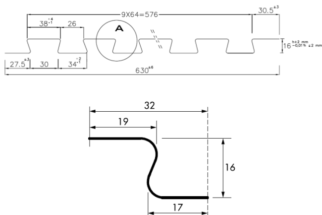
Fig. 1: – Afmetingen Lewis®-Zwaluwstaartplaten®
